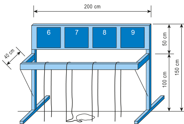
Obr. 10 - uzlový stojan
